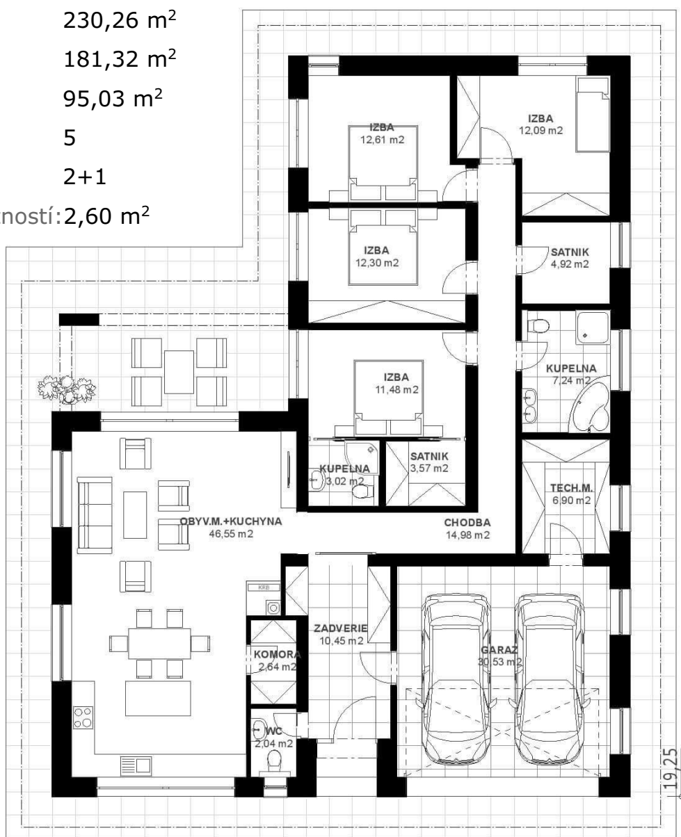
PÔDORYS 1.NP
