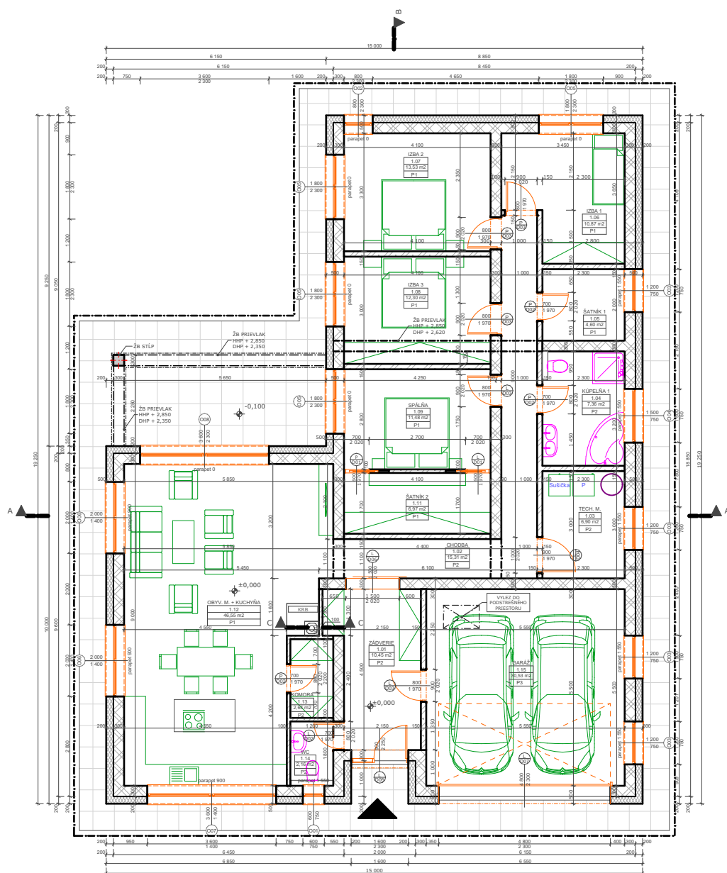
PÔDORYS 1.NP
